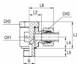
med B4-skärklämring
