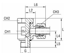
med B3-skärhylsa
