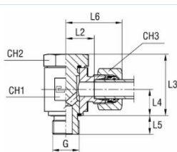
med B4-skärklämring
