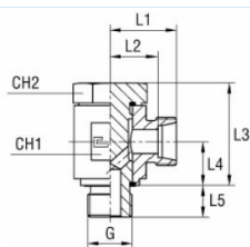
Grundkropp
