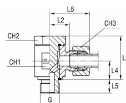
met B3-snijring
