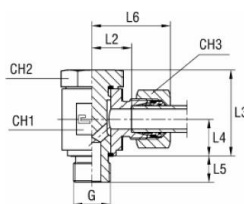
met B4-snijring
