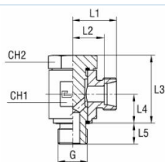
Osnovno tijelo
