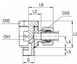
s řezným kroužkem B4
