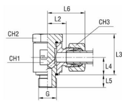
s řezným kroužkem B3
