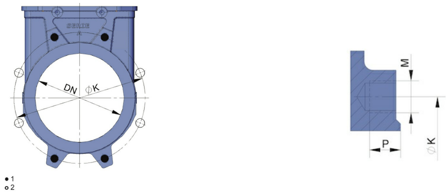
1...blind gat schroefdraad, 2...Doorlopende boring
