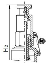
Päätykappale kaasutiivis tuuletuspainikkeella
