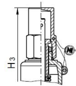
Päätykappale kaasutiivis suojakorkki
