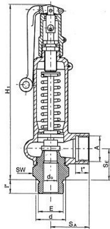
Päätykappale Ilmanpoistovipu kaasutiivis
