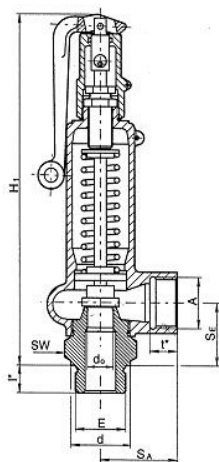
Κεφαλή Μοχλός εξαερισμού στεγανό στα αέρια
