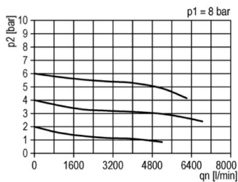
Diagramma di portata
