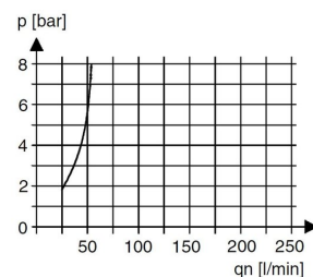
Olieforstøverens aktiveringsgrænse
