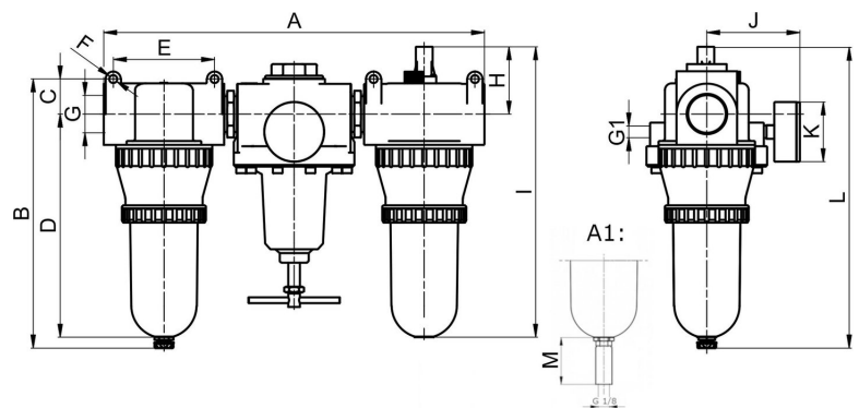
A1: supapă de purjare automată
