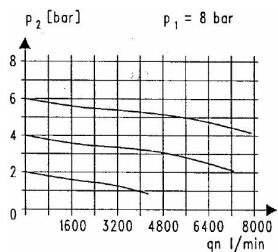
Virtauskaavio
