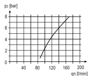
Öljysumuttimen toimintaraja
