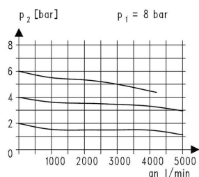
Virtauskaavio
