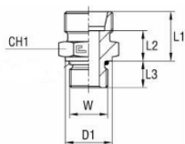
Grundkropp
