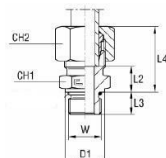
med B3-skärhylsa
