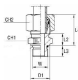
met B4-snijring
