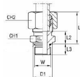
met B3-snijring
