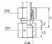
med B3-skärhylsa
