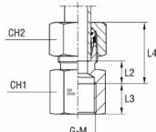
med B4-skärhylsa
