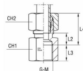
met B3-snijring
