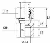
met B4-snijring
