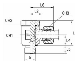
med B3-skärhylsa
