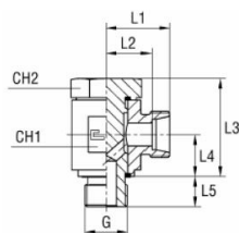
Grundkropp
