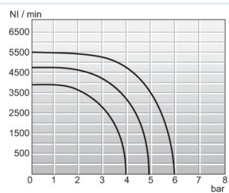
Διάγραμμα ροής 1/2"
