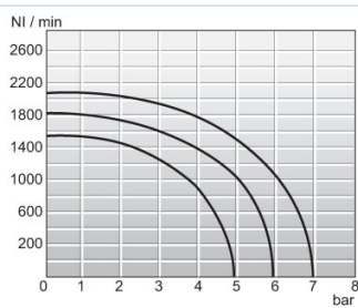
Διάγραμμα ροής 1/4"
