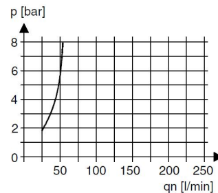
Öler-Ansprechgrenze
