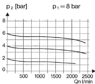
Durchflussdiagramm
