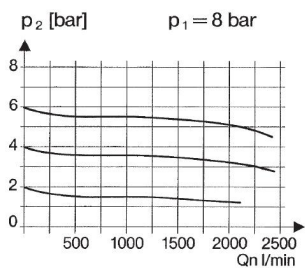
Průtokový diagramm
