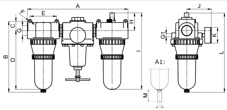
A1: automatisches Ablassventil
