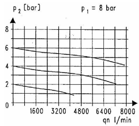
Durchflussdiagramm
