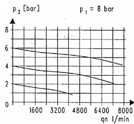
Průtokový diagramm
