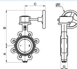
Wersja kołnierzowa
