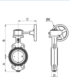
Zwischenflanschausführung
