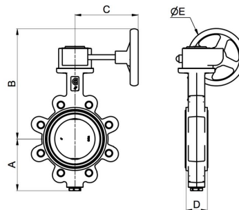
Prirubnička izvedba
