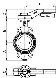
Meduflansna izvedba
