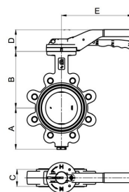
Přírubové provedení
