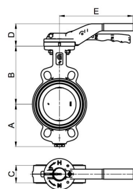
Mezipřírubové provedení
