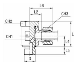
-val/-vel B3-vágógyűrűvel
