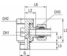
-val/-vel B4-vágógyűrűvel
