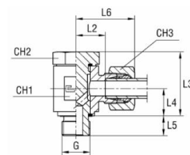
s řezným kroužkem B3
