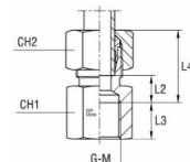
z pierścieniem zacinającym B3
