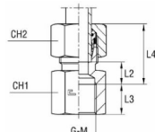
z pierścieniem tnącym B4
