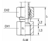
-val/-vel B3-vágógyűrűvel
