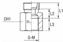
Grundkörper
