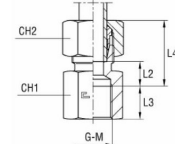
mit B3-Schneidring
