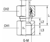
mit B4-Schneidring
