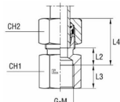
s řezným kroužkem B4
