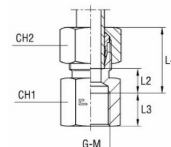
s řezným kroužkem B3
