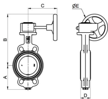
Zwischenflanschausführung
