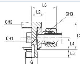
mit B3-Schneidring
