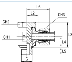
mit B4-Schneidring
