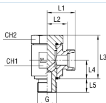
Grundkörper
