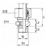
z pierścieniem tnącym B4
