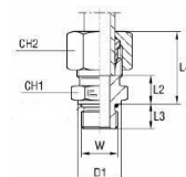
z pierścieniem zacinającym B3
