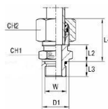
mit B4-Schneidring
