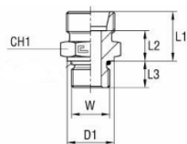
Grundkörper
