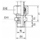
mit B4-Schneidring
