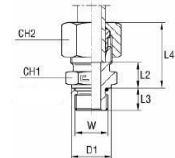
mit B3-Schneidring
