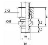
mit B3-Schneidring
