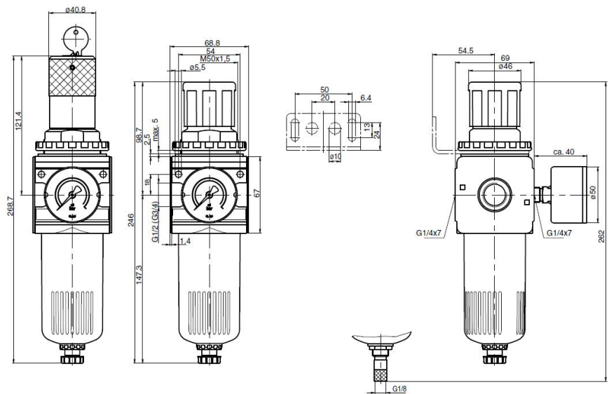
halbautomatisches Ablasventil
