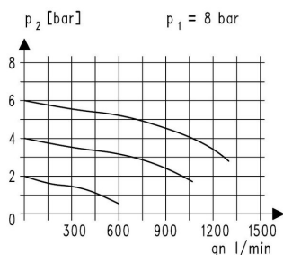
Wykres przepływu
